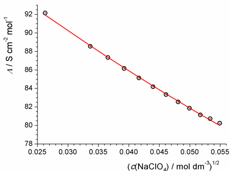
Slika 30. Ovisnost molarne provodnosti \text{NaClO}_4 o njegovoj koncentraciji u smjesi otapala \text{MeOH}/\text{CH}_2\text{Cl}_2 ( \varphi = 0,5 ); \vartheta = (25,0 \pm 0,1)^\circ\text{C} .
