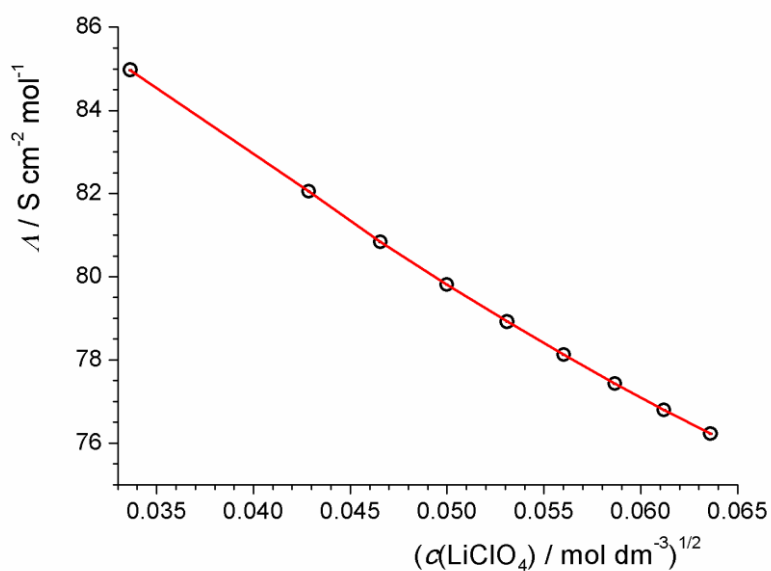
Slika 29. Ovisnost molarne provodnosti \text{LiClO}_4 o njegovoj koncentraciji u smjesi otapala \text{MeOH}/\text{CH}_2\text{Cl}_2 ( \varphi = 0,5 ); \vartheta = (25,0 \pm 0,1)^\circ\text{C} .
