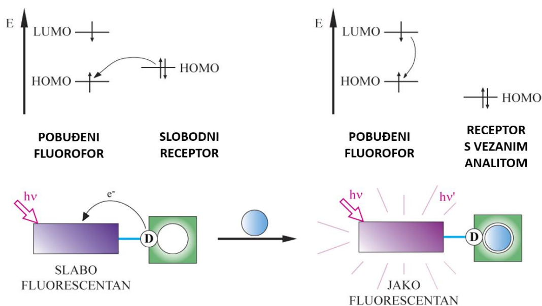
Slika 57. Pojačanje fluorescencije inhibicijom fotoinduciranog prijenosa elektrona vezanjem kationa.
