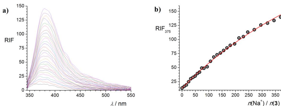
Slika 78. a) Fluorimetrijska titracija spoja 3 ( c = 1,47 \times 10^{-6} \text{ mol dm}^{-3} ) s \text{NaClO}_4 ( c = 3,022 \times 10^{-3} \text{ mol dm}^{-3} ) u smjesi otapala \text{MeOH}/\text{CH}_2\text{Cl}_2 ( \varphi = 0,5 ); \vartheta = (25,0 \pm 0,1) ^\circ\text{C} ; V_0(\mathbf{3}) = 2,5 \text{ cm}^3 ; \lambda_{\text{ex}} = 333 \text{ nm} ; širine pukotina: ulazna 5 nm, izlazna 7,5 nm; l = 1 \text{ cm} . Spektri su korigirani za razrjeđenje. b) Ovisnost relativnog intenziteta fluorescencije otopine spoja 3 pri 375 nm o omjeru množina dodanog \text{NaClO}_4 i spoja 3 . \circ eksperimentalne vrijednosti; — izračunane vrijednosti.
