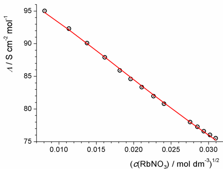
Slika 32. Ovisnost molarne provodnosti \text{RbNO}_3 o njegovoj koncentraciji u smjesi otapala \text{MeOH}/\text{CH}_2\text{Cl}_2 ( \varphi = 0,5 ); \vartheta = (25,0 \pm 0,1)^\circ\text{C} .
