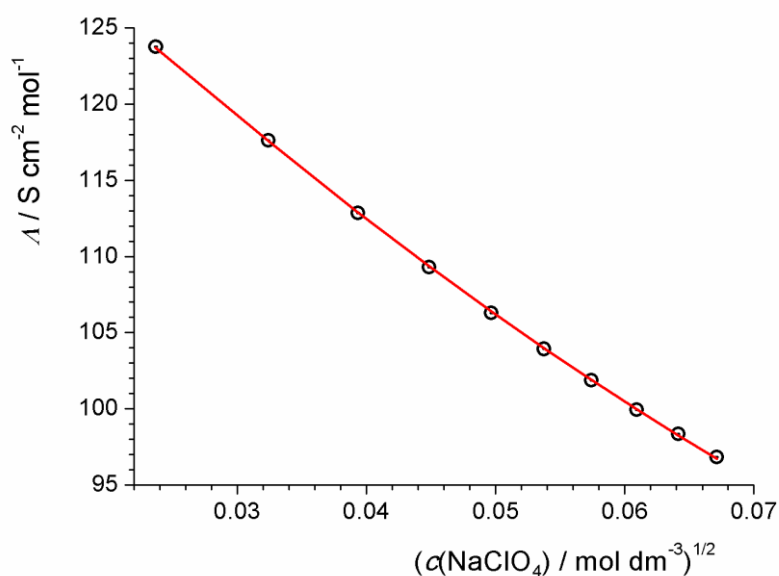
Slika 28. Ovisnost molarne provodnosti \text{NaClO}_4 o njegovoj koncentraciji u smjesi otapala \text{MeCN}/\text{CH}_2\text{Cl}_2 ( \varphi = 0,5 ); \vartheta = (25,0 \pm 0,1)^\circ\text{C} .
