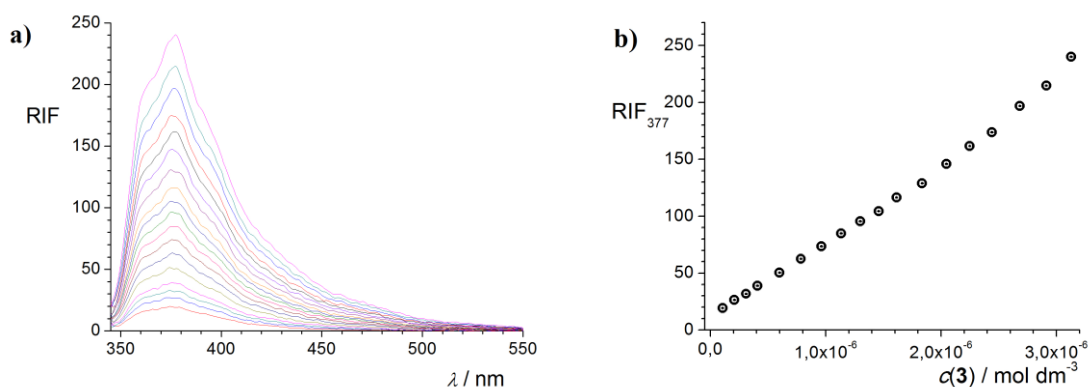
Slika 53. a) Ovisnost emisijskih spektara spoja 3 u smjesi otapala \text{MeCN}/\text{CH}_2\text{Cl}_2 ( \varphi = 0,5 ) o njegovoj koncentraciji; \vartheta = (25,0 \pm 0,1) ^\circ\text{C} ; V_0 = 2,5 \text{ cm}^3 ; \lambda_{\text{ex}} = 333 \text{ nm} ; širine pukotina: ulazna 7,5 nm, izlazna 7,5 nm; l = 1 \text{ cm} . b) Ovisnost relativnog intenziteta fluorescencije otopine spoja 3 pri 377 nm o njegovoj koncentraciji.
