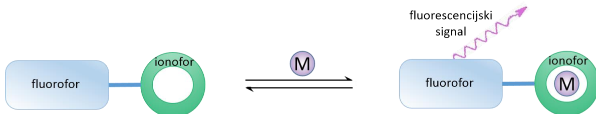
Slika 13. Ilustracija principa rada fluorescentnog kationskog senzora.
