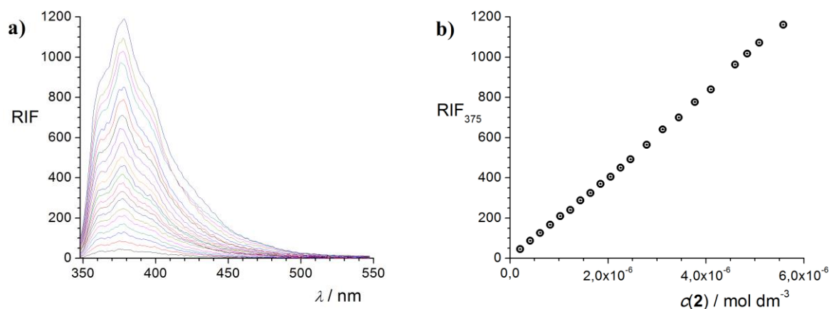
Slika 65. a) Ovisnost emisijskih spektara spoja 2 u smjesi otapala MeOH/CH 2 Cl 2 ( \varphi = 0,5 ) o njegovoj koncentraciji; \vartheta = (25,0 \pm 0,1) ^\circ\text{C} ; V_0 = 2,5 \text{ cm}^3 ; \lambda_{\text{ex}} = 333 \text{ nm} ; širine pukotina: ulazna 5 nm, izlazna 7,5 nm; l = 1 \text{ cm} . b) Ovisnost relativnog intenziteta fluorescencije otopine spoja 2 pri 375 nm o njegovoj koncentraciji.
