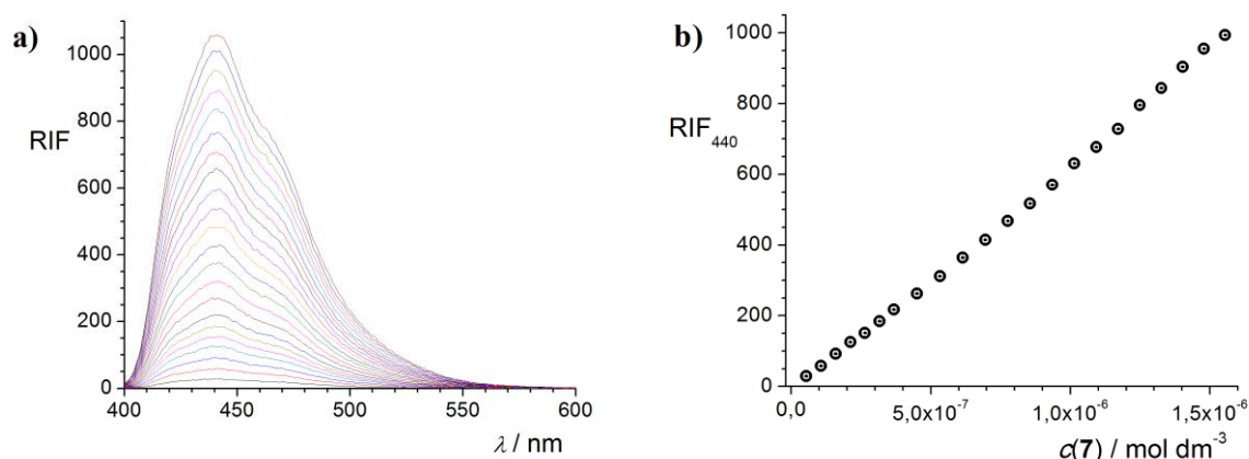
Slika 98. a) Ovisnost emisijskih spektara spoja 7 u smjesi otapala MeCN/CH 2 Cl 2 ( \varphi = 0,5 ) o njegovoj koncentraciji; \vartheta = (25,0 \pm 0,1)^\circ\text{C} ; V_0 = 2,5\text{ cm}^3 ; \lambda_{\text{ex}} = 386\text{ nm} ; širine pukotina: ulazna 7 nm, izlazna 3 nm; l = 1\text{ cm} . b) Ovisnost relativnog intenziteta fluorescencije otopine spoja 7 pri 440 nm o njegovoj koncentraciji.
