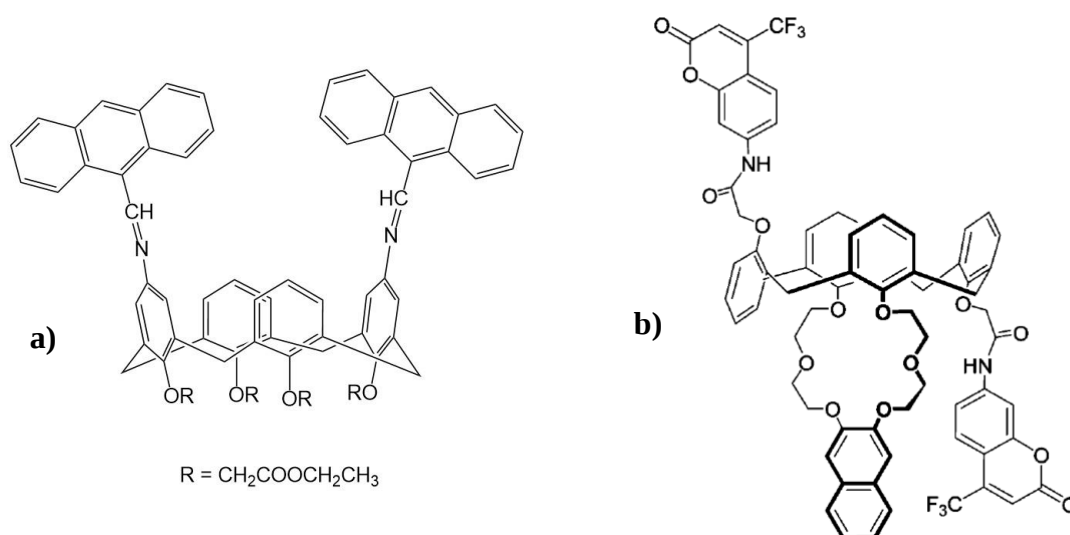
Slika 14. Primjeri fluorescentnih kaliksarenskih senzora temeljenih na:
