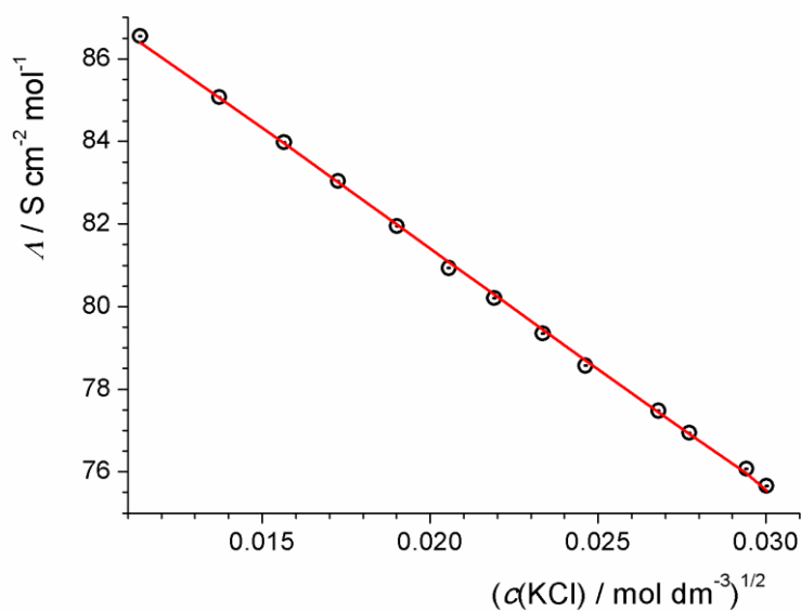
Slika 31. Ovisnost molarne provodnosti \text{KCl} o njegovoj koncentraciji u smjesi otapala \text{MeOH}/\text{CH}_2\text{Cl}_2 ( \varphi = 0,5 ); \vartheta = (25,0 \pm 0,1)^\circ\text{C} .
