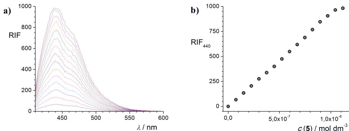
Slika 109. a) Ovisnost emisijskih spektara spoja 5 u smjesi otapala MeOH/CH 2 Cl 2 ( \varphi = 0,5 ) o njegovoj koncentraciji; \vartheta = (25,0 \pm 0,1)^\circ\text{C} ; V_0 = 2,5 \text{ cm}^3 ; \lambda_{\text{ex}} = 404 \text{ nm} ; širine pukotina: ulazna 5 nm, izlazna 2,5 nm; l = 1 \text{ cm} . b) Ovisnost relativnog intenziteta fluorescencije otopine spoja 5 pri 440 nm o njegovoj koncentraciji.
