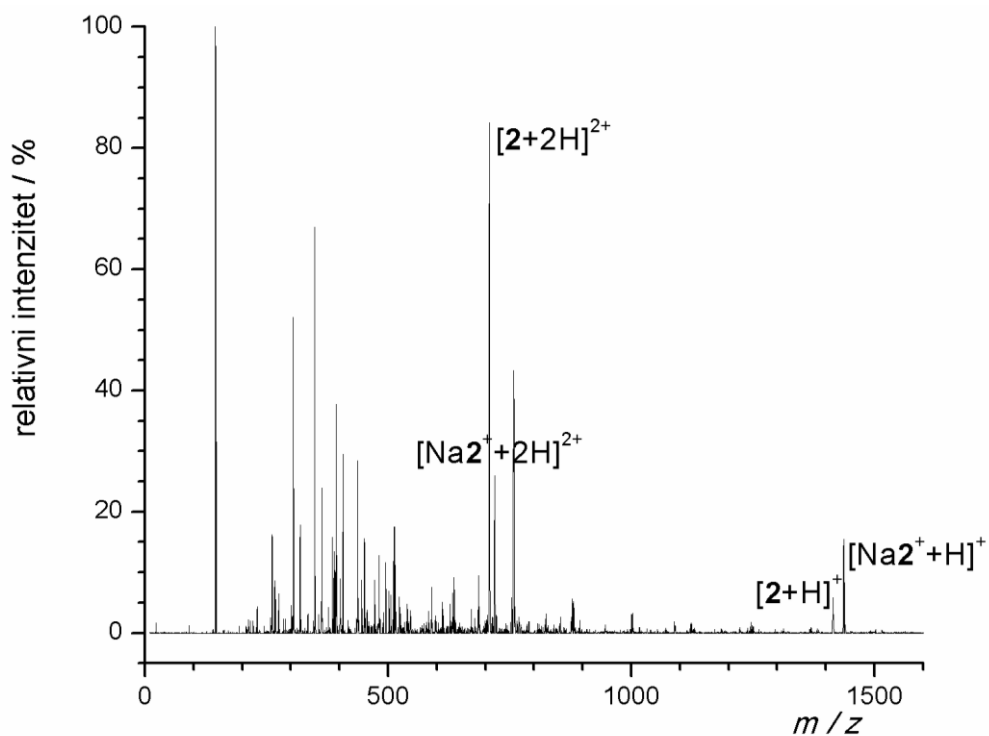
Slika 73. Maseni spektar kompleksa \text{Na}^{2+} u smjesi otapala MeOH/CH 2 Cl 2 ( \varphi = 0,5 ).
