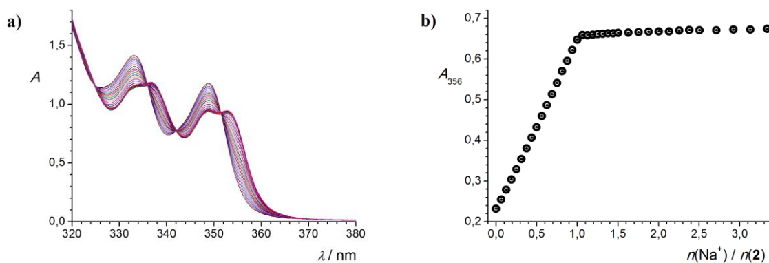
Slika 38. a) Spektrofotometrijska titracija spoja 2 ( c = 1,51 \times 10^{-4} \text{ mol dm}^{-3} ) s \text{NaClO}_4 ( c = 2,51 \times 10^{-3} \text{ mol dm}^{-3} ) u smjesi otapala \text{MeCN}/\text{CH}_2\text{Cl}_2 ( \varphi = 0,5 ); \vartheta = (25,0 \pm 0,1)^\circ\text{C} ; V_0(\mathbf{2}) = 2,0 \text{ cm}^3 ; l = 1 \text{ cm} . Spektri su korigirani za razrjeđenje. b) Ovisnost apsorbancije otopine spoja 2 pri 356 nm o omjeru množina dodanog \text{NaClO}_4 i spoja 2 .
