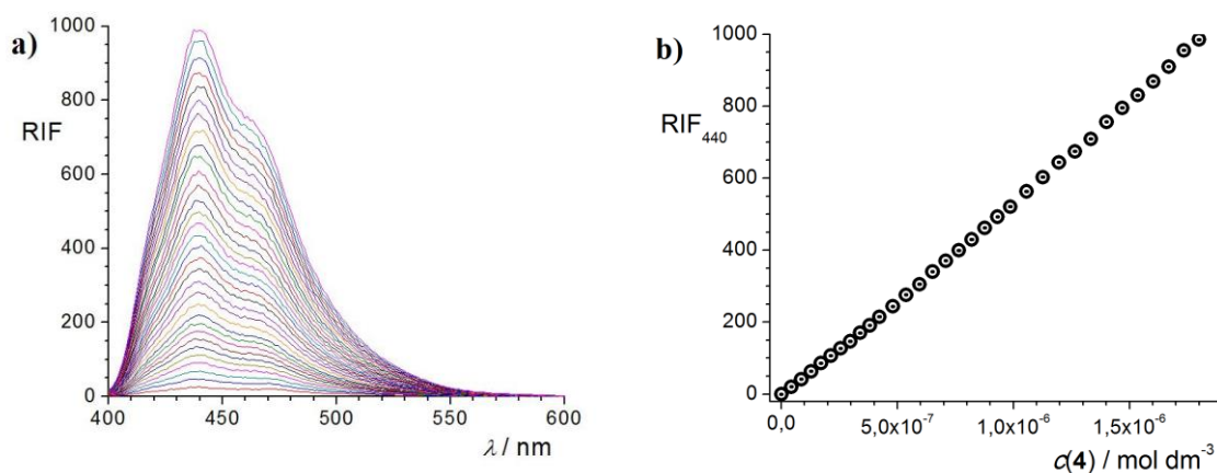
Slika 82. a) Ovisnost emisijskih spektara spoja 4 u smjesi otapala MeCN/CH 2 Cl 2 ( \varphi = 0,5 ) o njegovoj koncentraciji; \mathcal{S} = (25,0 \pm 0,1) ^\circ\text{C} ; V_0 = 2,5 \text{ cm}^3 ; \lambda_{\text{ex}} = 386 \text{ nm} ; širine pukotina: ulazna 7 nm, izlazna 3 nm; l = 1 \text{ cm} . b) Ovisnost relativnog intenziteta fluorescencije otopine spoja 4 pri 440 nm o njegovoj koncentraciji.
