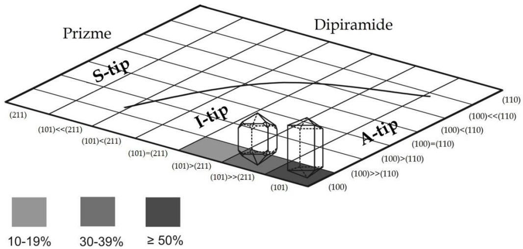
Slika 4.7: Zastupljenost pojedinih tipova cirkona prikazano na modificiranom Pupinovom dijagramu (PUPIN, 1980; BALEN et al., 2014) uz prikaz područja rasprostranja pojedinih tipova granita (S – sedimentnog podrijetla; I – magmatskog; A – anorogenog).
