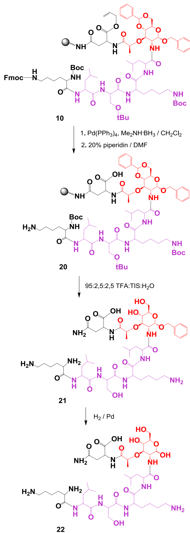
Shema 9. Sinteza nezaštićenog linearnog glikopeptida \text{H-N}^c\text{-Lys-Leu-Ser-Lys-Leu-Mur-Asn-OH} ( 22 )
