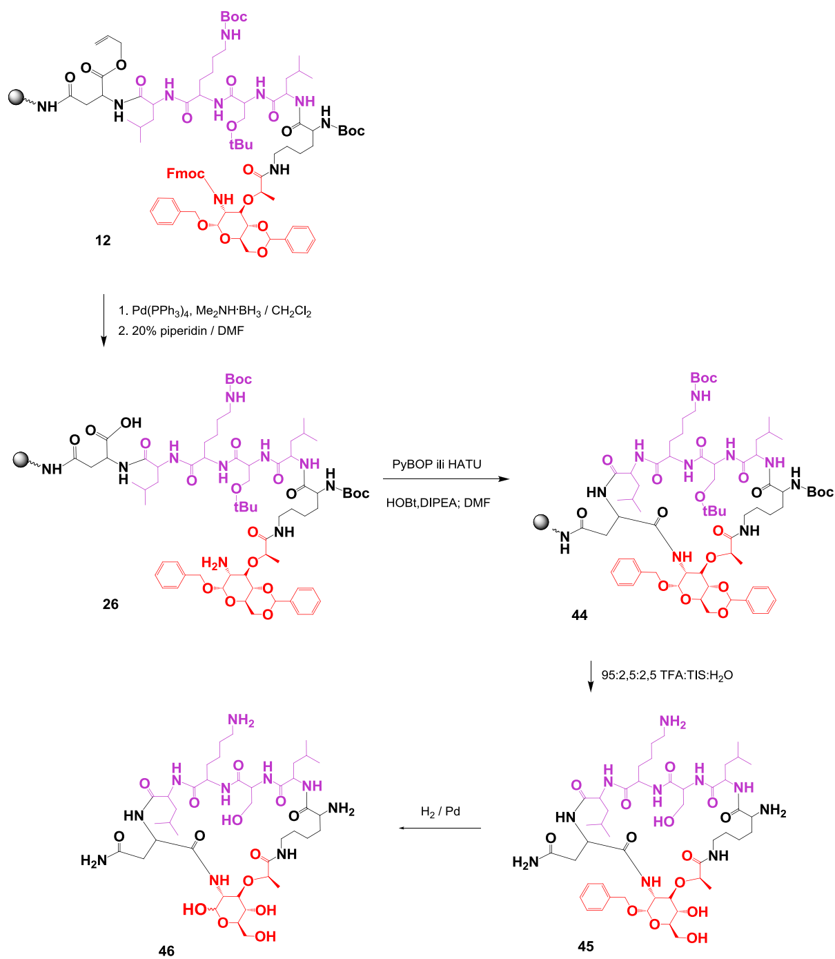
Shema 19. Sinteza nezaštićenog cikličkog glikopeptida ciklo[Mur- N c -Lys-Leu-Ser-Lys-Leu-Asn] ( 46 )
