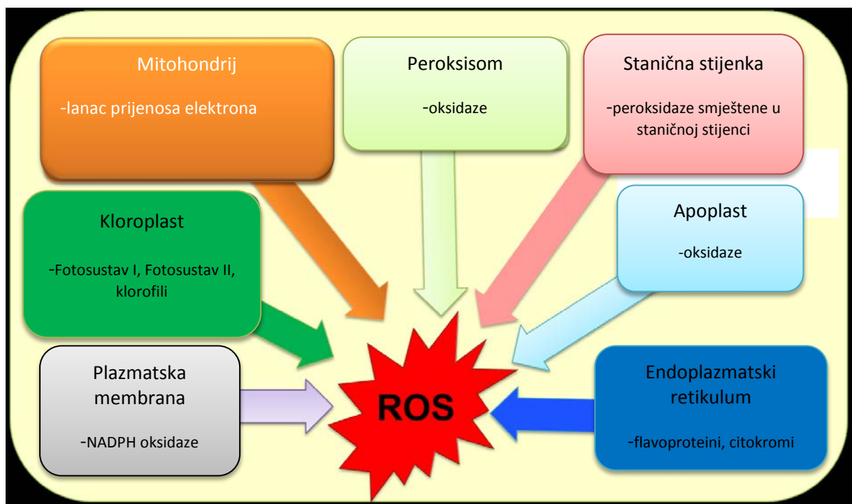
Slika 2. Mjesta proizvodnje ROS u biljci (preuzeto i prilagođeno iz Hasanuzzaman i sur., 2013b)
