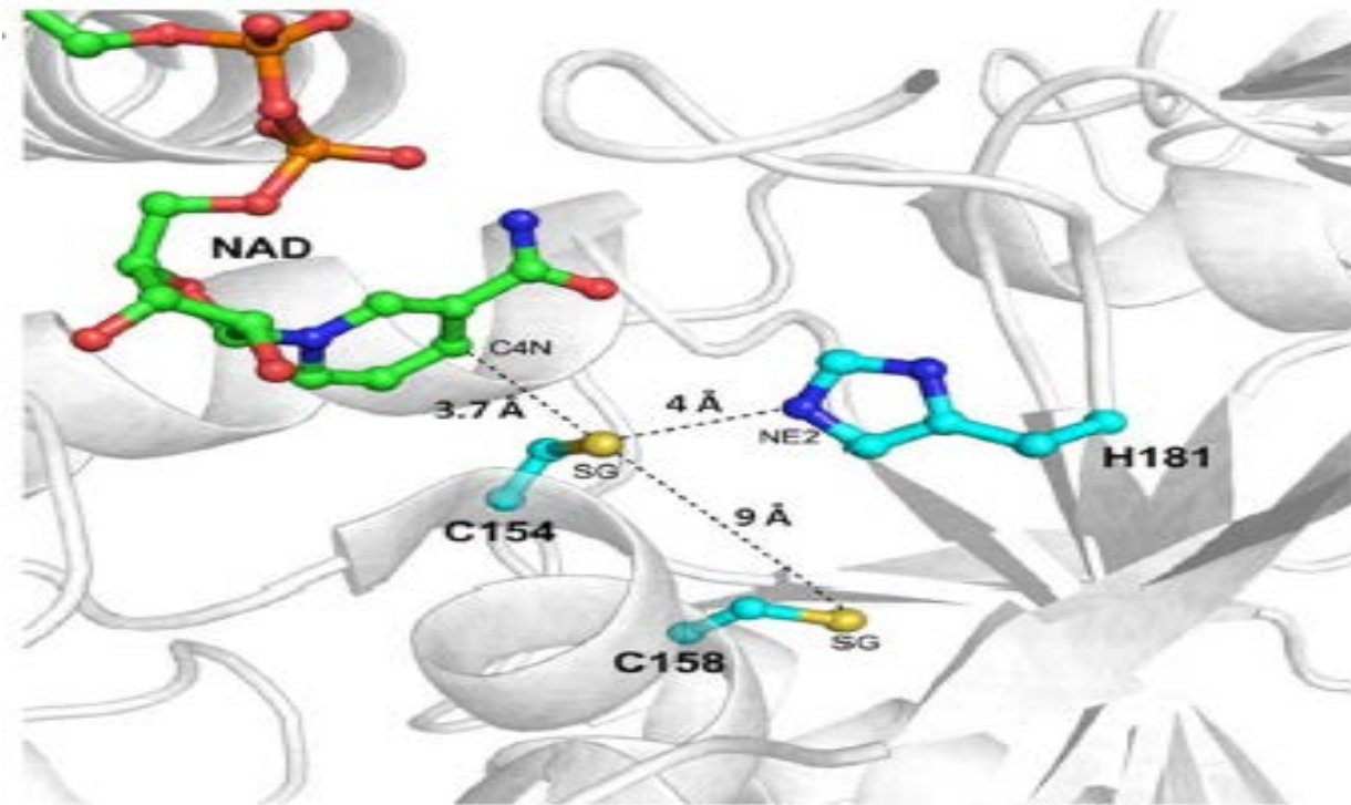
Slika 1.: Kristalna struktura katalitičkog mjesta citoplazmatske GAPDH iz riže ( Oryza sativa ) sa vezanim kofaktorom \text{NAD}^+ . Bojom su posebno istaknuti bočni ogranaci Cys-154 i His-181 koji su bitni za katalizu te bočni ogranak Cys-158. (preuzeto iz Zaffagnini i sur. 2013)
