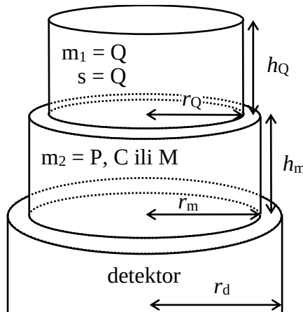
Slika 4.6 Prikaz geometrije ( g = 2 ) za tri mjerenja koja daju ulazne parametre za određivanje \mu_M i \mu_C pomoću MC simulacija. Za sva tri mjerenja s = Q i m_1 = Q , dok se m_2 mijenja, tj. kod prvog mjerenja m_2 = P (prazna posuda, zrak), kod drugog m_2 = C (matrica uzorka C) i kod trećeg m_2 = M (matrica uzorka M).
