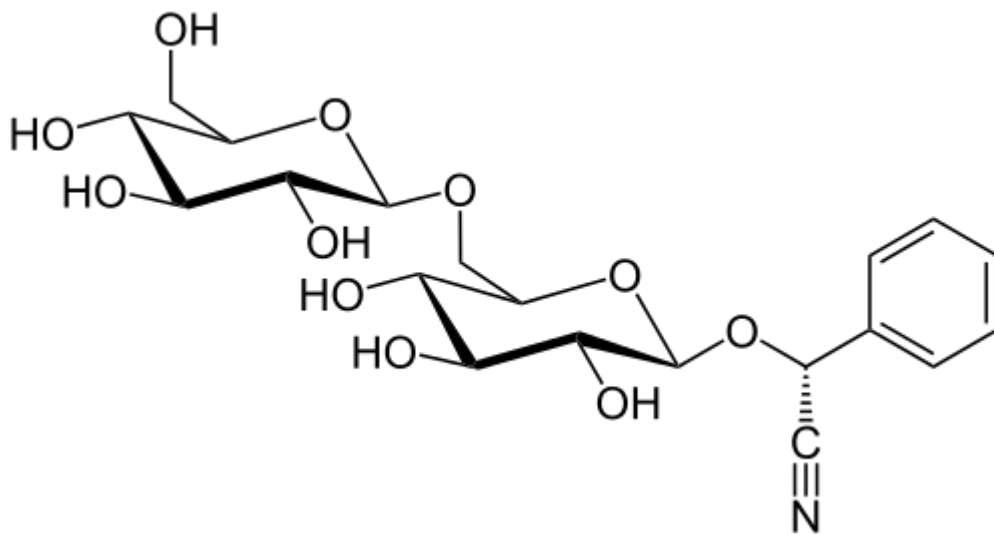
Slika 6: Amigdalinalin, cijanogeni glikozid nađen u gorkim bademima,
