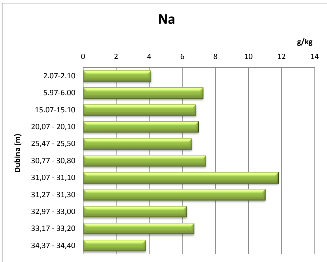
Slika 47. Koncentracija natrija
