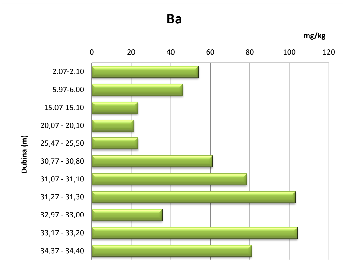
Slika 57. Koncentracija barija
