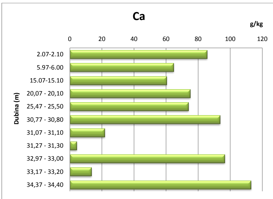
Slika 42. Koncentracija kalcija
