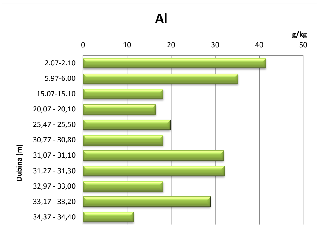
Slika 41. Koncentracija aluminija
