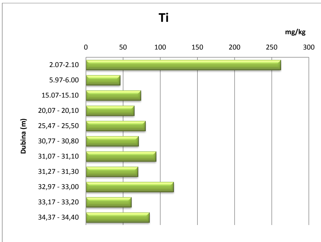
Slika 58. Koncentracija titana
