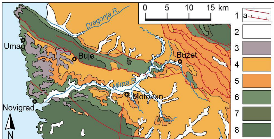
Slika 2. Geološka karta SZ Istre; 1. Rasjed, 2. Naslage kvartara (uglavnom holocen), 3. Terra rossa (holocen), 4. Fliš (eocen), 5. Liburnijske naslage, foraminiferski vapnenac i prijelazne naslage (paleocen?, eocen), 6. Rudistni vapnenac (kreda), 7. Dolomiti i breče (kreda), 8. Vapnenac i dolomit (jura) (FELJA i sur., 2015)
