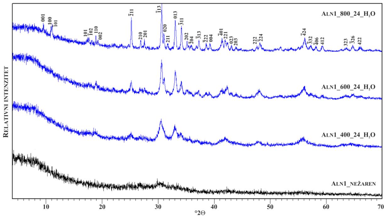
Slika 10. Usporedni difraktogrami nežarenog te hidrotermalno tretiranog uzorka ALN1 kroz 24 h na 400, 600 i 800°C
