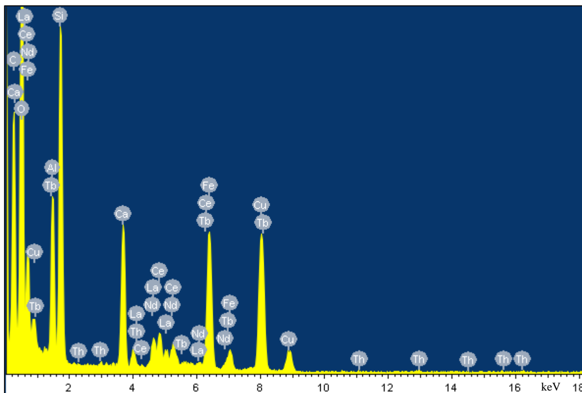
Slika 89. Reprezentativni EDS spektar uzorka ALN1
