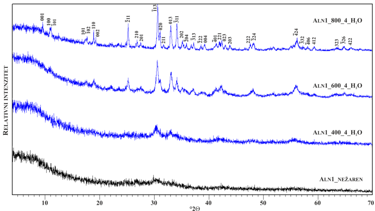
Slika 9. Usporedni difraktogrami nežarenog te hidrotermalno tretiranog uzorka ALN1 kroz 4 h na 400, 600 i 800°C
