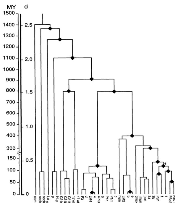
Slika 7. Filogenetsko stablo 34 proteina citokroma P450. ♦ predstavljaju događaj duplikacije gena. Neoznačena mjesta granjanja predstavljaju događaje specijacije. „*“ predstavljaju pretpostavljenu duplikaciju gena, iz razloga što je prerano reći o razilaženju dvije vrste (Preuzeto iz Nelson i Strobel, 1987).
