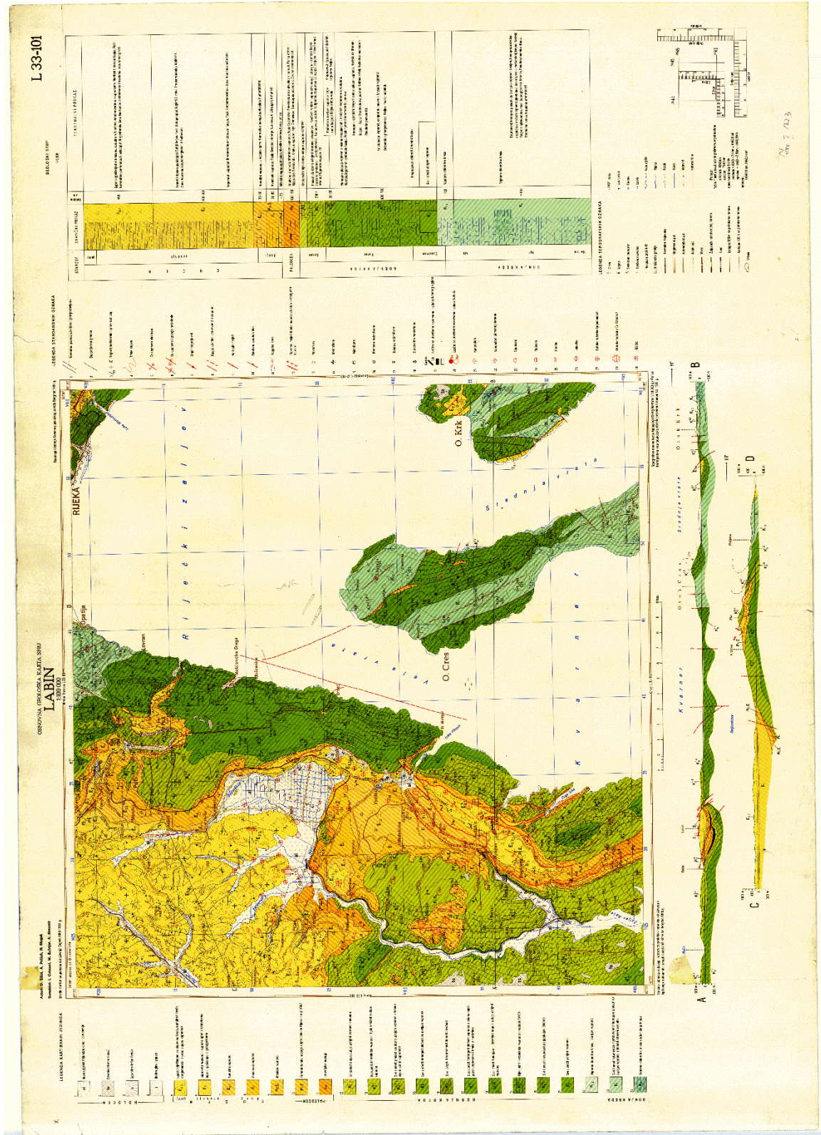
Prilog 1 Osnovna geološka karta SFRJ - List Labin
