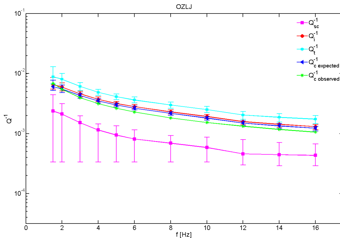
Slika A.13 Rezultati za postaju OZLJ. Q^{-1} -faktori u ovisnosti o frekvenciji dobiveni MLTWA metodom te mjereni Q_c^{-1} observed preuzet iz Dasović (2015). Prikazane su i pripadajuće standardne devijacije dobivene za parove Le^{-1} i B_0 područja 68% pouzdanosti F-distribucije.
