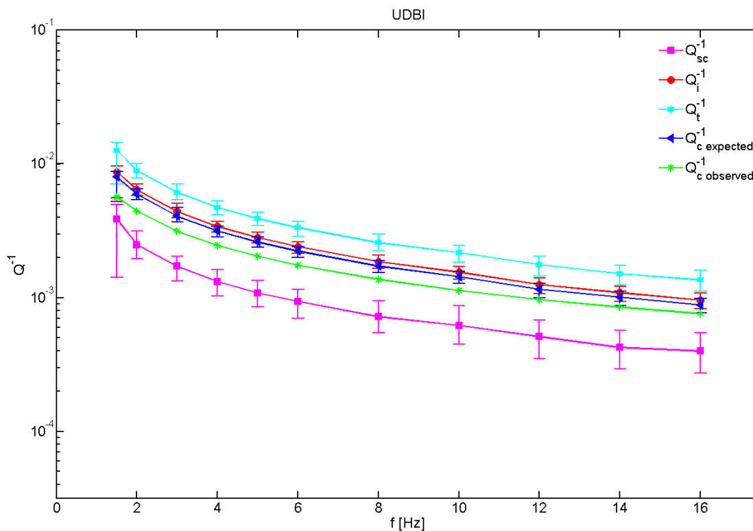
Slika A.14 Rezultati za postaju UDBI. Q^{-1} -faktori u ovisnosti o frekvenciji dobiveni MLTWA metodom te mjereni Q_c^{-1} observed preuzet iz Dasović (2015). Prikazane su i pripadajuće standardne devijacije dobivene za parove Le^{-1} i B_0 područja 68% pouzdanosti F-distribucije.
