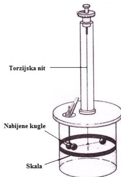
Slika 2.1: Postav Coulombovog eksperimenta.
