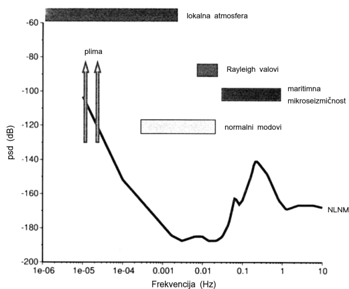
Slika 3.5 Dominantni izvori seizmičkih šumova na vertikalnim sensorima (gravimetrima i seizmometrima) zajedno s novim modelom niskog šuma (engl. new low-noise model , NLNM, Peterson, 1993). Izvori šuma spomenuti na slici stvaraju ograničenja u detekciji malih signala normalnih modova. Preuzeto iz Widmer-Schmidrig (2003).
