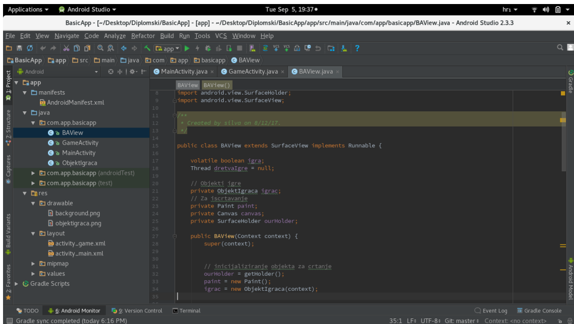
Slika 5.5: BAView.java
