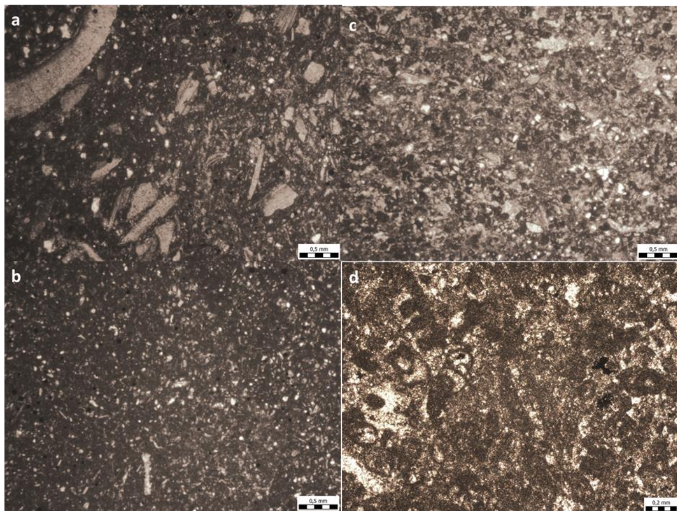
Slika 16. a, b – mikrofacijes prve jedinice turona; c – mikrofacijes druge jedinice turona; d – mikrofacijes treće jedinice turona.
