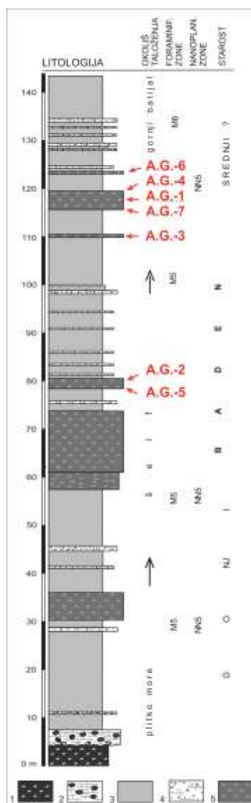
Slika 4.1.1. Geološki stup snimljenog profila s označenim mjestima uzorkovanja (crvene oznake), Legenda: 1- metagabro, 2- algalni vapnenac, 3- lapor, 4- bioklastični vapnenac, 5- tuf (preuzeto iz KOVAČIĆ i sur., 2015)
