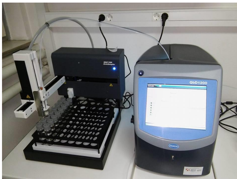
Slika 8. Autosampler a) injektiranje H_3PO_4 u uzorke; b) ekran s prikazom detekcije CO_2 signala; d) cijeli prikaz analizatora za određivanje ugljika u tekućim uzorcima.
