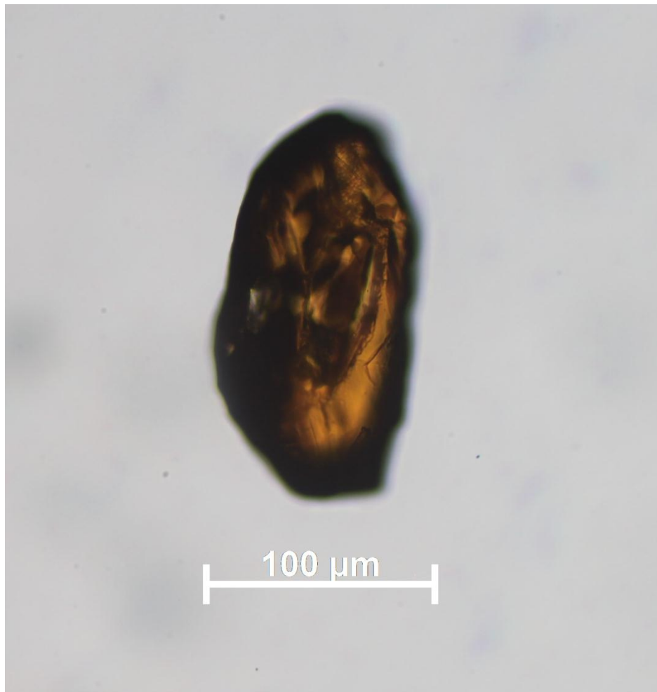
Slika 18. Uzorak MR-6, rutil bez uključenog analizatora
