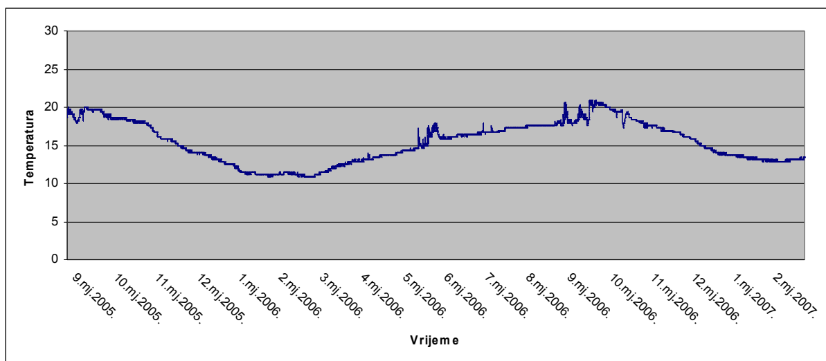
Slika 11. - Profil temperature u ulaznom dijelu jame kod Iškog Mrtovnjaka, na 10,5 m dubine
