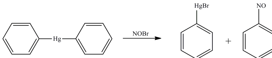
Slika 7. Sinteza nitrozobenzena.
