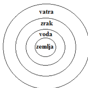
Slika 10.: Slika sublunarnog područja u idealnom slučaju
