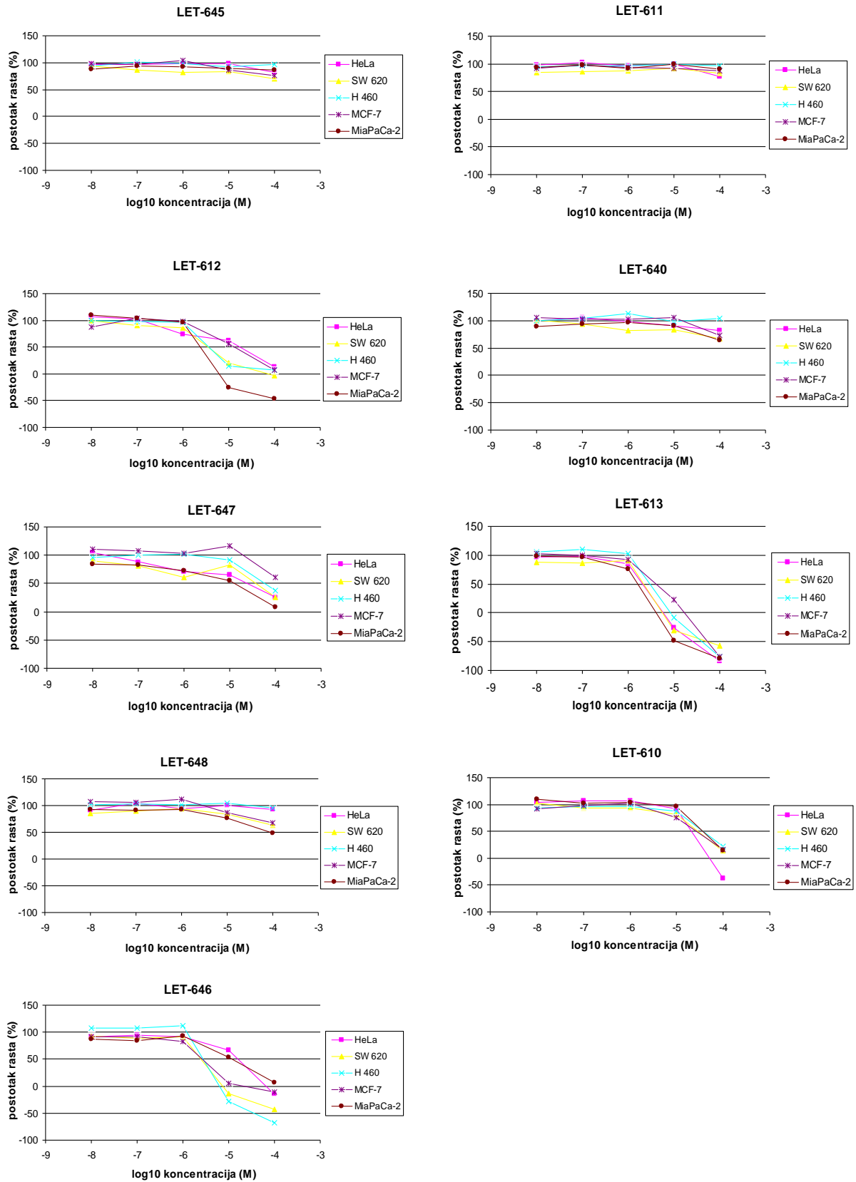
Slika 11. Utjecaj makrocikličkih spojeva u koncentracijama 10 -4 M do 10 -8 M na rast tumorskih stanica navedenih linija HeLa, SW620, H460, MCF-7 i MiaPaCa-2 u uvjetima in vitro . Prikazane su krivulje ovisnosti postotka rasta stanica o koncentraciji spoja.
