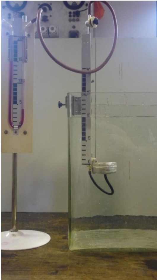
Slika 4.18. Hidrostatski tlak u tekućini
