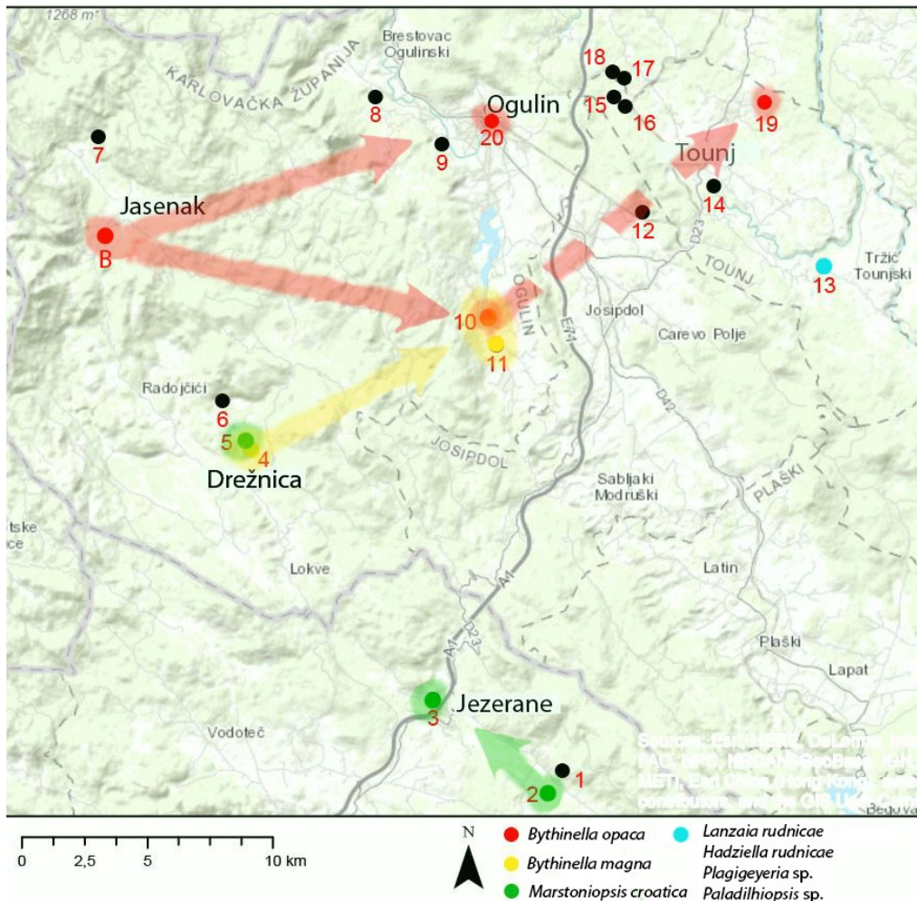
Slika 56. Rasprostranjenost svojiti Bythinella opaca , Bythinella magna , Marstoniopsis croatica , Lanzaia rudnicae , Hadziella rudnicae , Plagigeyeria sp. i Paladilhopsis sp. te pretpostavka povezanosti populacija na temelju hidrogeološke karte
