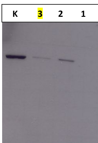
Slika 3.13. Western analiza s anti-GST protutijelima. K -kontrola, GST-ArgRS; 3 -uzorak C, kompleks GST-ArgRS i His 6 -SerRS je zadržan na kuglicama jer se GST-ArgRS vezao na njih, signal daje GST-ArgRS; 2 -uzorak B, GST-ArgRS koji se vezao na kuglice; 1 -uzorak A, His 6 -SerRS se nije vezao na kuglice jer nema GST tag te nema signala.
