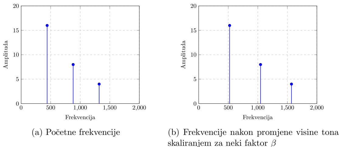
Slika 3.5: Promjena visine tona iz frekvencijske perspektive
