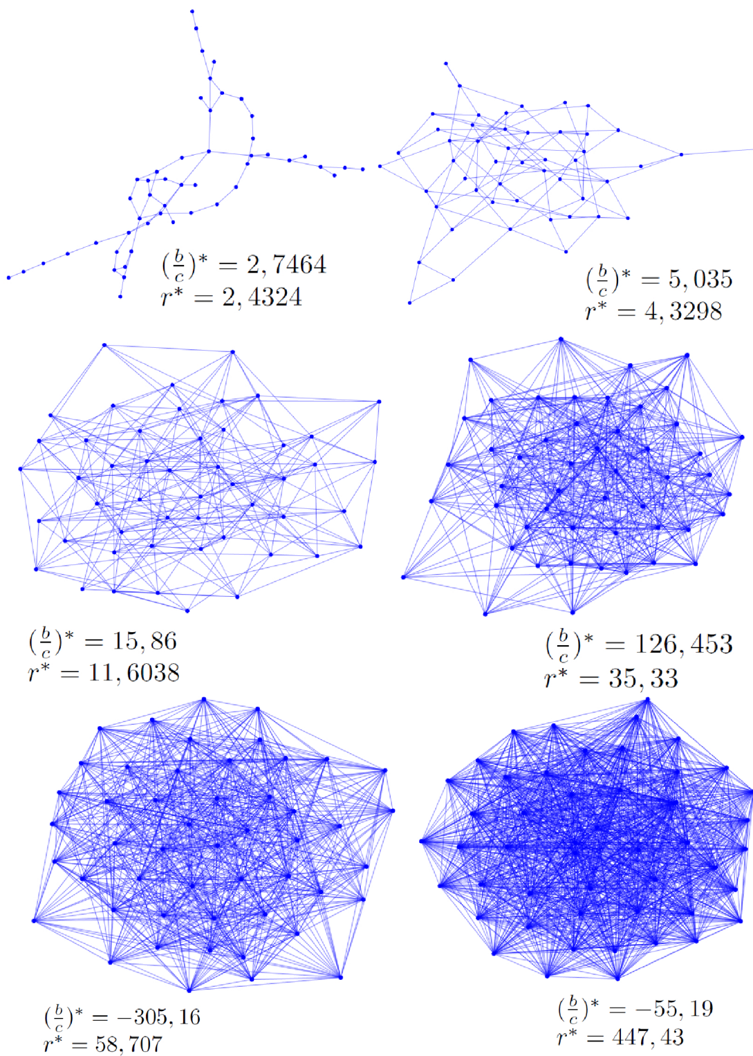
Slika 6.10: Mreže s N = 50 vrhova i njihove vrijednosti \left(\frac{b}{c}\right)^* i r^*
