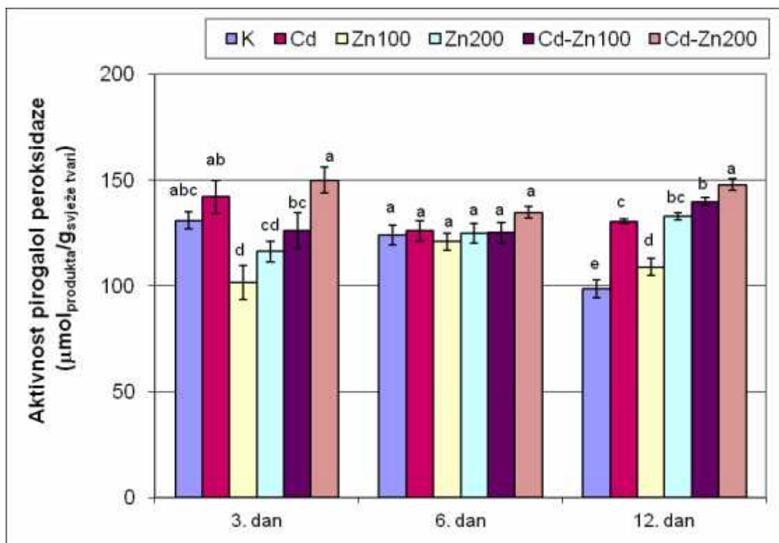
Slika 6. Aktivnost pirogallol peroksidaze u ekstraktima vodene le e 3, 6, 12. dana (K – kontrola; Cd –uzorak s 10 \mu M Cd; Zn 100 – uzorak s 100 \mu M Zn; Zn 200 – uzorak s 200 \mu M Zn; Cd-Zn 100 – uzorak s 10 \mu M Cd i 100 \mu M Zn; Cd-Zn 200 – uzorak s 10 \mu M Cd i 100 \mu M Zn). Rezultati su prikazani kao srednja vrijednost od 8 replika \pm standardna pogreška. Vrijednosti prikazane stupcima ozna enim razli itim slovima se statisti ki zna ajno razlikuju ( P < 0.05 ).
