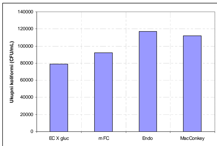
Slika 20. Broj ukupnih koliforma dobiven nacjepljivanjem uzorka vode (Vugrov potok, postaja 1) na četiri različite podloge za izolaciju koliformnih bakterija: EC X Gluc agar, m-Faecal Coliform agar, Endo agar i MacConkey agar
