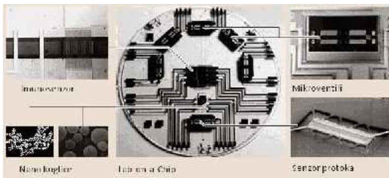
Slika 4.1. Laboratorij-na- čipu. Na slici se mogu vidjeti mikrokanali koji vode tekućinu do mikrouređaja za analizu. Ovaj čip služi za imunodetekciju s magnetnim kuglicama koje služe za fiksaciju i detekciju antigena. Preuzeto iz Springer Handbook of Nanotechnology, 2004.
