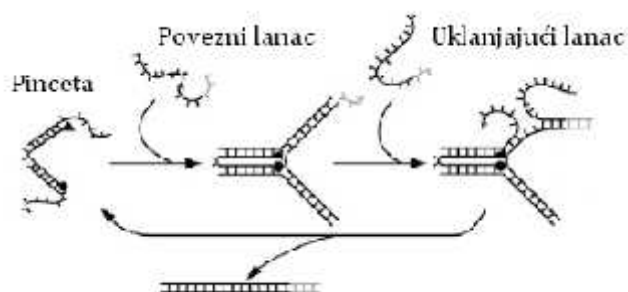
Slika 1.1. Optička se pinceta zatvara i otvara pomoću poveznih (prvi korak) i uklanjajućih (drugi korak) lanca. Povezni i uklanjajući lanci su komplementarni lanci i nakon opuštanja pincete izlaze iz sustava. Preuzeto i prilagođeno iz Liedl i sur. 2007.
