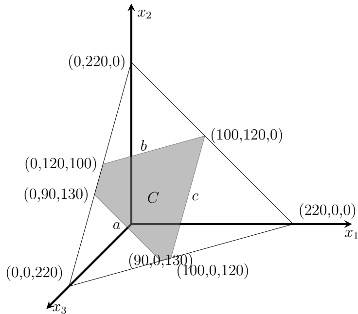
Slika 1.3: Rješenje problema gradova
