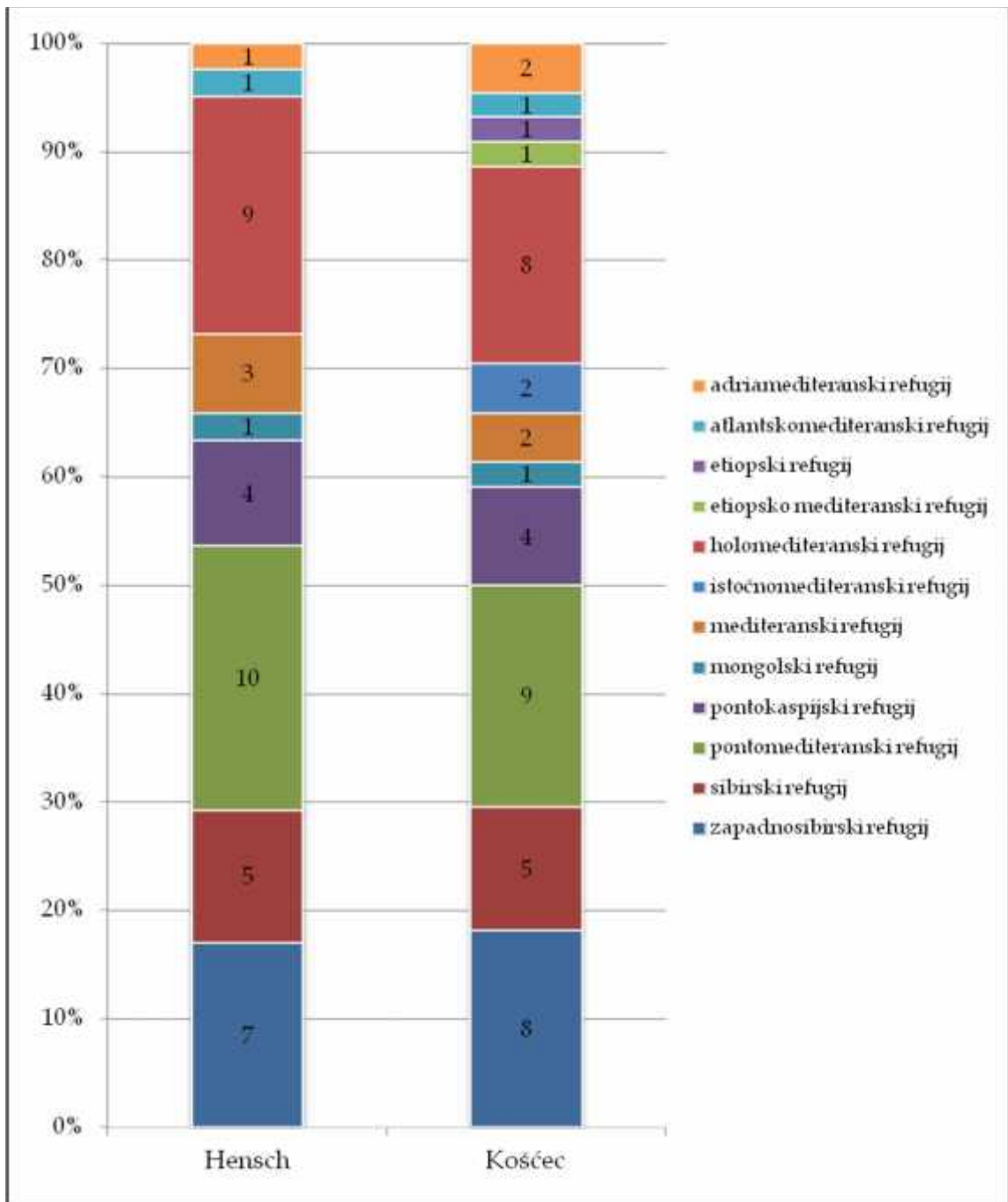
Slika 64: Usporedba zbirke Hensch i Košćec prema porijeklu faune vretenaca (Dévai 1976).
