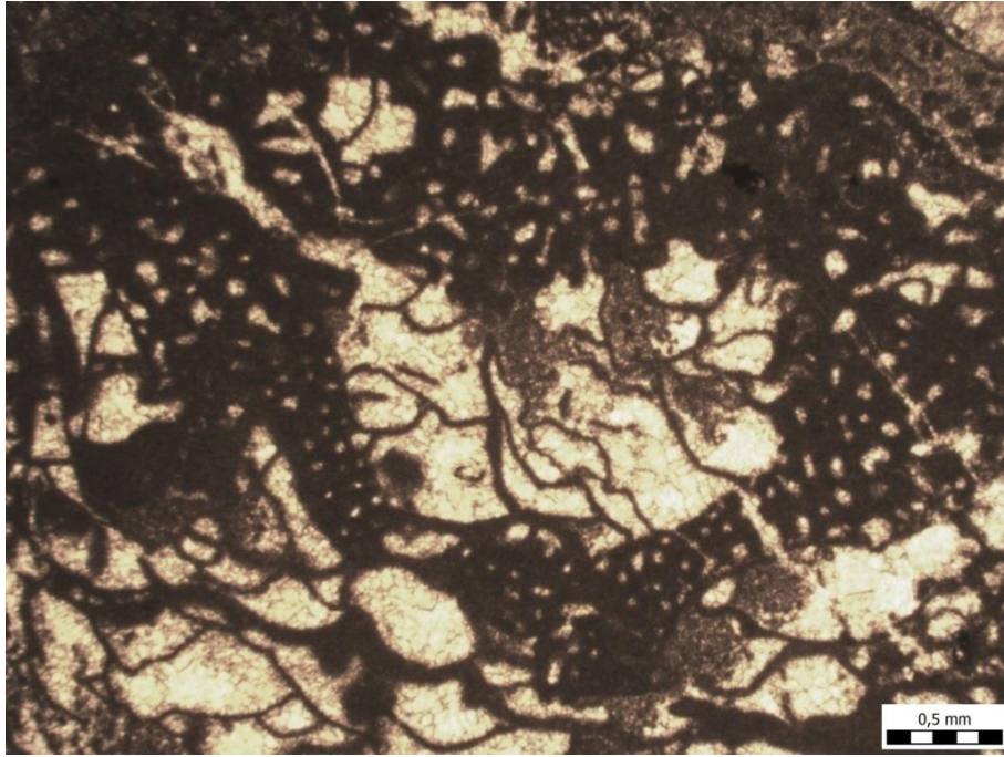
Slika 5.3.4. Mikrofacijesni tip (MF3) bačinski flintston donjoaptske starosti.
