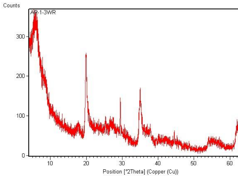
Slika 5.4. Rendgenogram ukupnog mineralnog sastava uzorka AR3.
