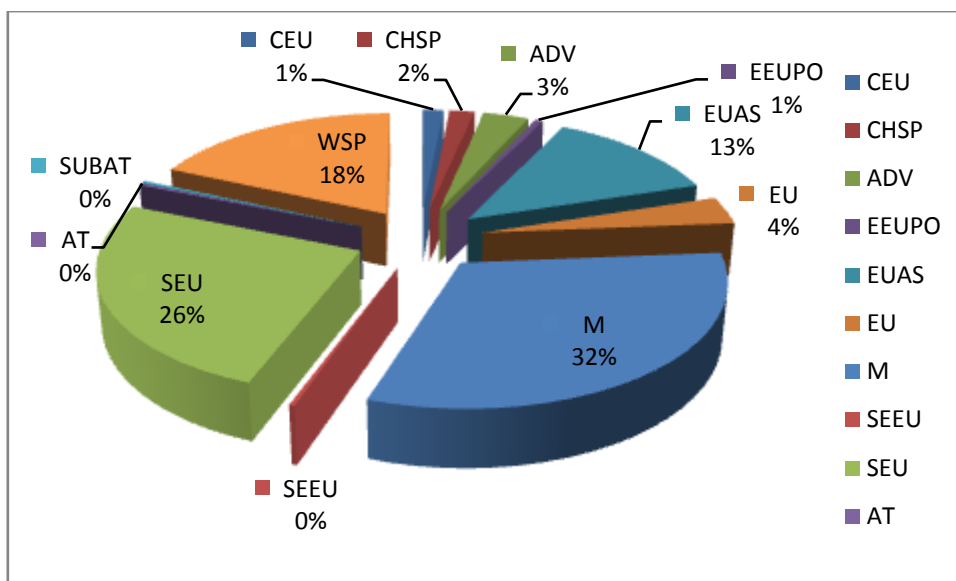
Slika 18. Spektar florinih elemenata (podelementi nisu uključeni)
