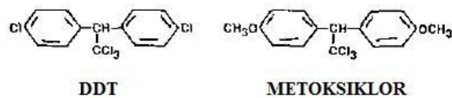
Slika 8. Strukturni prikaz molekule diklordifeniltrikloretana (DDT-a) i metoksiklora. (Prilagođeno na temelju Reuber, 1980.)
