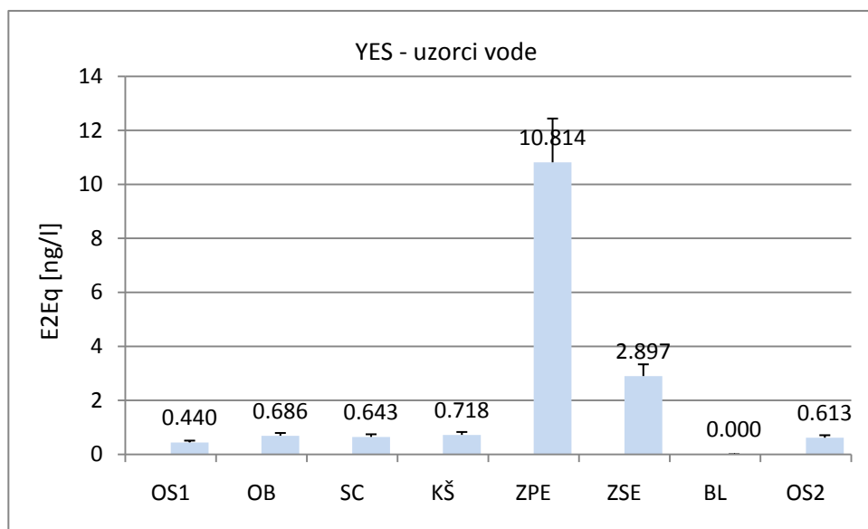
Slika 13. Vrijednosti E2Eq uzoraka vode (OS1– Otok Samoborski, OB – Oborovo, SC – Sisak Crnac, KŠ – Košutarica, ZSE- sekundarni ispušt, ZPE – primarni ispušt, BL – kontrola, OS2 – preliminarni uzorak Otok Samoborski).
