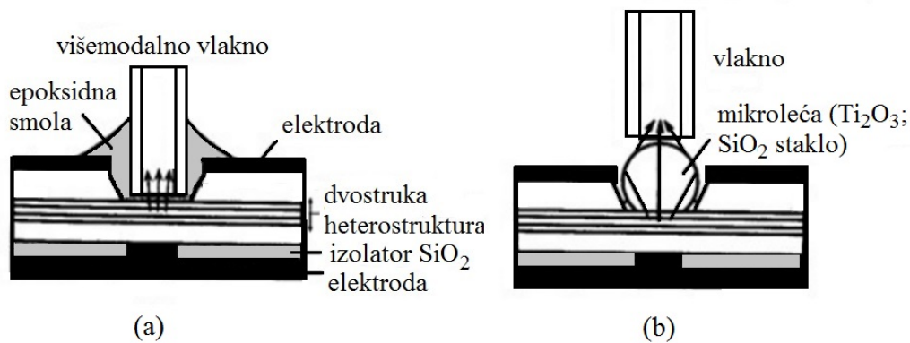
Slika 5.4: Tehnika povezivanja svjetleće diode s površinskom emisijom svjetlosti s optičkim vlaknom: (a) pomoću epoksidne smole, (b) pomoću mikroleće [13].
