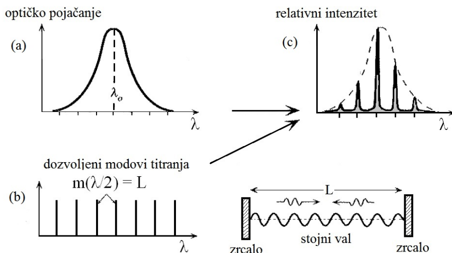
Slika 4.7: (a) Graf optičkog pojačanja u ovisnosti o valnoj duljini. (b) Dozvoljeni modovi titranja ovise od duljini optičkog rezonatora. (c) Izlazni spektar [13].
