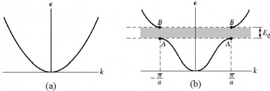
Slika 2.3: Graf ovisnosti energije elektrona o valnom vektoru za: (a) elektrone u prvokutnoj potencijalnoj jami, (b) elektrone u periodičkom potencijalu kristalne rešetke konstante a [6].
