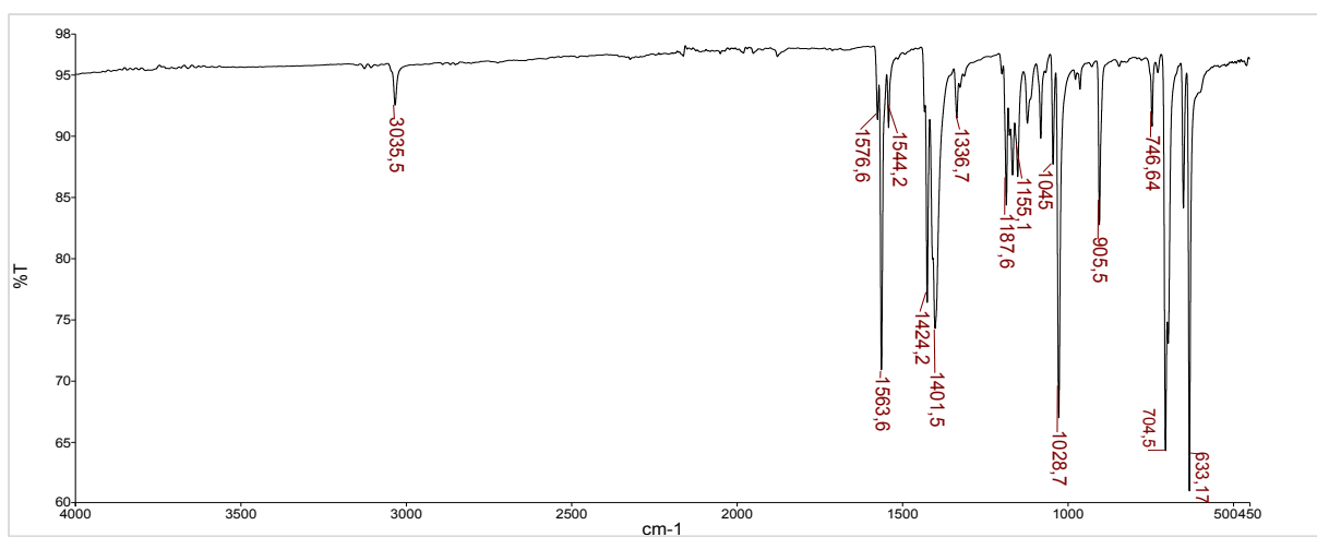
Slika D5. IR spektar spoja [\text{CdI}_2(5\text{-Brpm})_2]_n (5).
