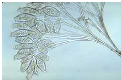
Slika 9. Opercularia sp.
