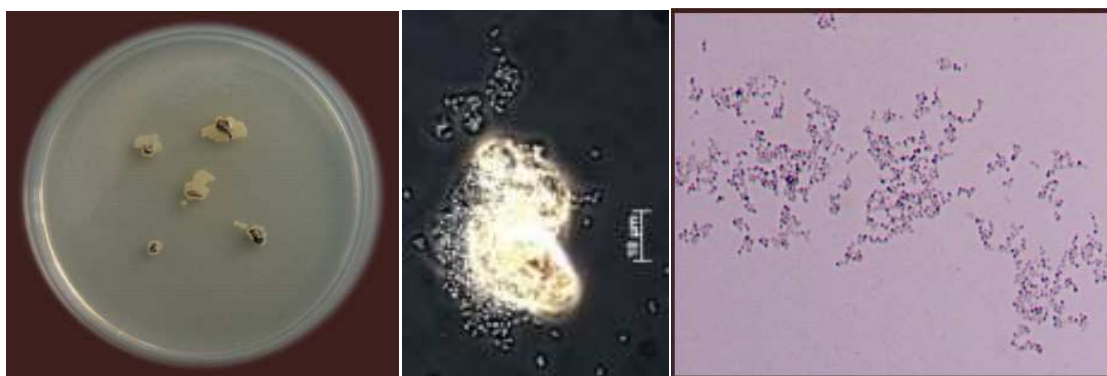
Slika 5. (1) Acinetobater junii uzgojena oko čestica zeolitnog tufa, (2) stanice A. junii imobilizirane na zeolitnom tufu, (3) plava zrnca polifosfata u stanicama A. junii , (Hrenović i sur. 2009.)
