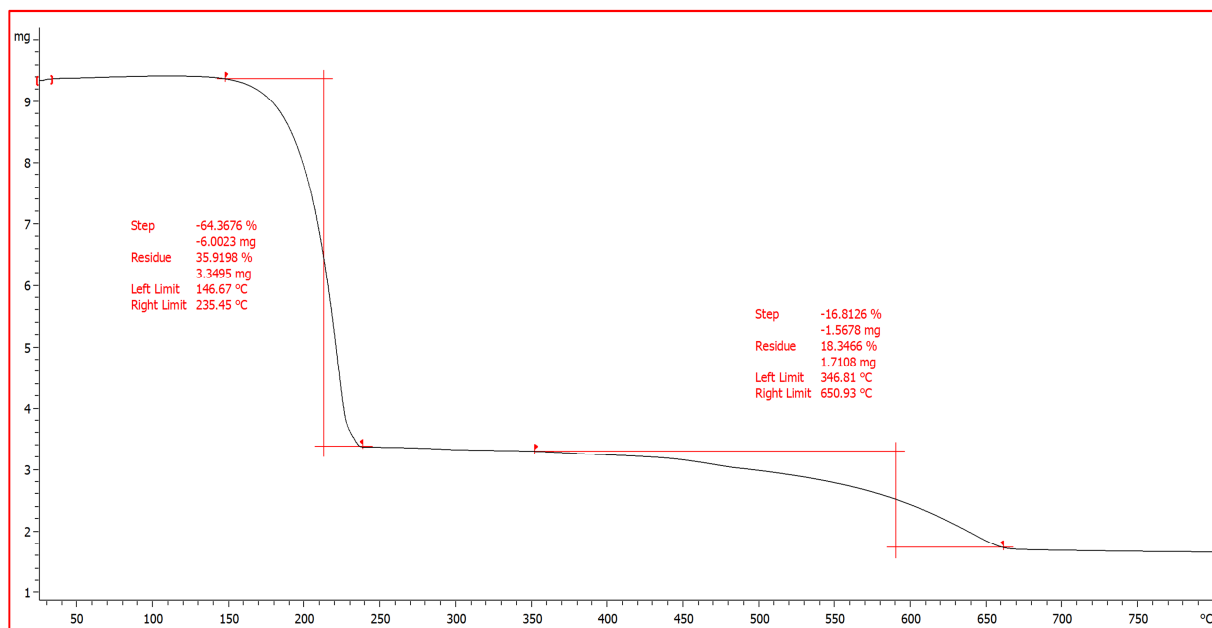
Slika 36. TGA krivulja spoja [CuBr 2 (Cl-pz) 2 ] (4).
