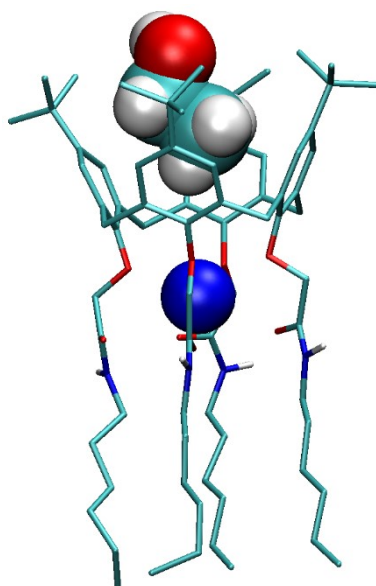
Slika 46: Struktura adukta \text{Na}^+ - \text{EtOH} u etanolu pri 25\text{ }^\circ\text{C} . Vodikovi atomi vezani na ugljikove atome izostavljeni su radi jasnoće prikaza.
