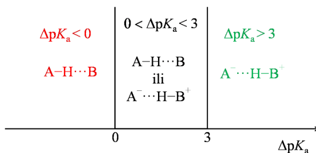
Slika 2.6. Shematski prikaz empirijskog pravila temeljenog na razlici vrijednosti pK_a za predviđanje nastajanja soli i kokristalâ.
