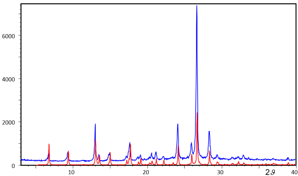
Slika 7.6. Difraktogrami praškastog uzorka 2-metilpiridinijevog N -(2-karboksifenil)hidrogenglicinata; plavo – izmjereni, crveno – računati.
