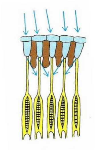
Slika 18. Općeniti shematski prikaz dijela superpozicijskog oka. (Zoology, 1991.)
