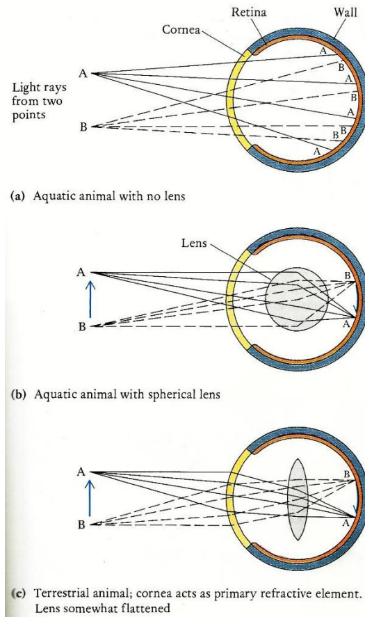
Slika 5. U oku vodenih životinja bez leće (a) zrake svjetlosti iz izvora A i B ne konvergiraju, već daju više točaka na retini, pa ne dolazi do stvaranja slike. Sferična leća vodenih životinja (b) uzrokuje lom svjetlosti tako da svaka zraka daje po jednu točku, stvarajući tako sliku. U kopnenih životinja (c) rožnica djeluje kao glavna površina za lom svjetlosti, a spljoštenija leća služi samo za precizno fokusiranje.
