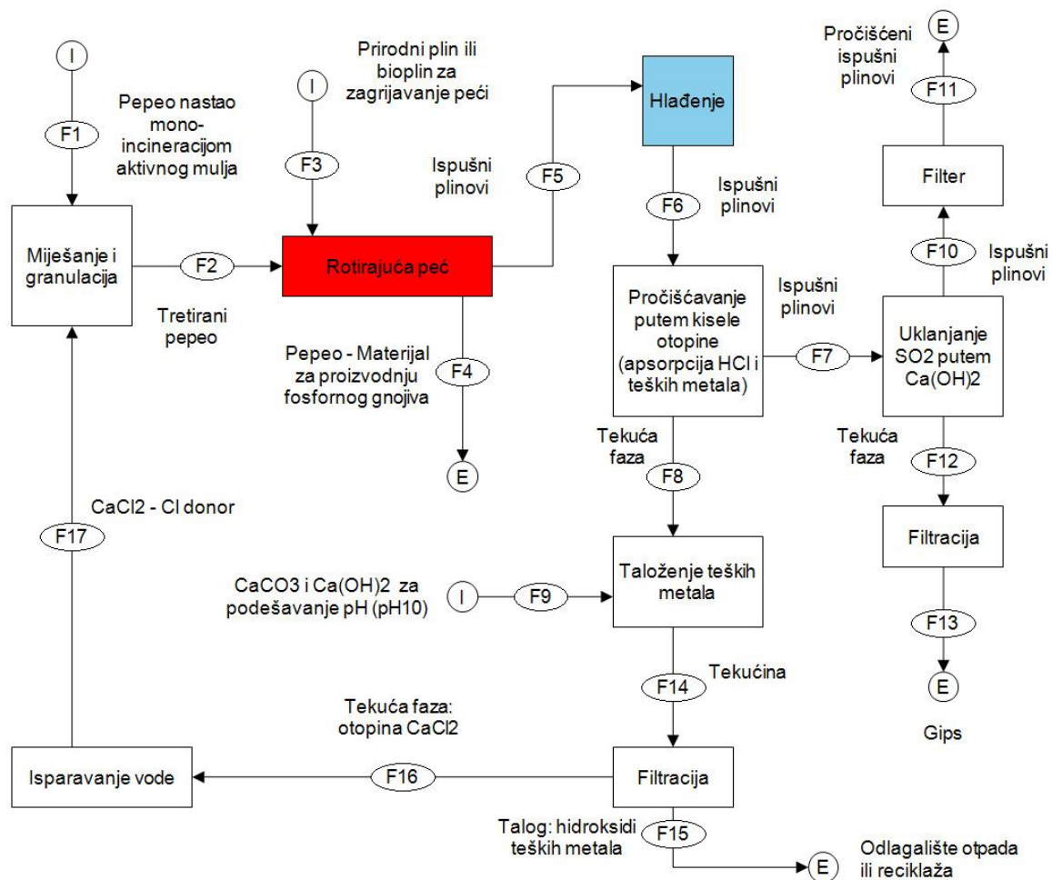
Slika 13: Shema elemenata SUSAN-tehnologije s naglaskom na pročišćavanje ispušnih plinova izrađena u STAN-sofveru na temelju skice g. Adama iz BAM-a.
