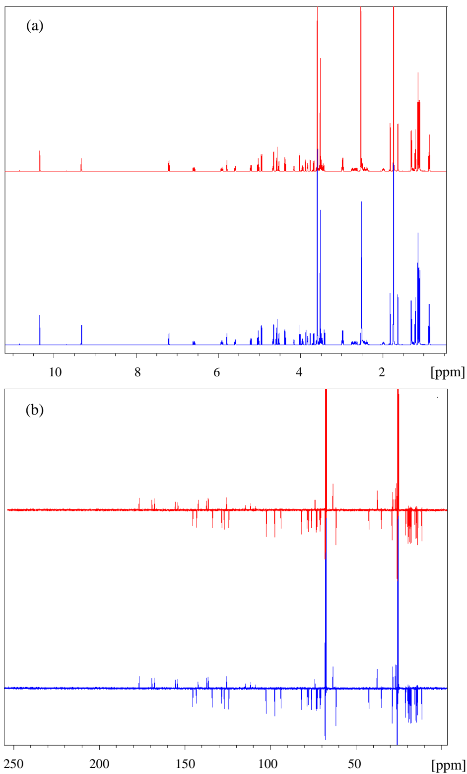
Slika 63. Spektri ^1\text{H} (a) i DEPTq (b) NMR za Fdx u THF- d_8 bez dodatka iona kalcija (plavo) i nakon dodatka \text{CaCl}_2 (crveno)
