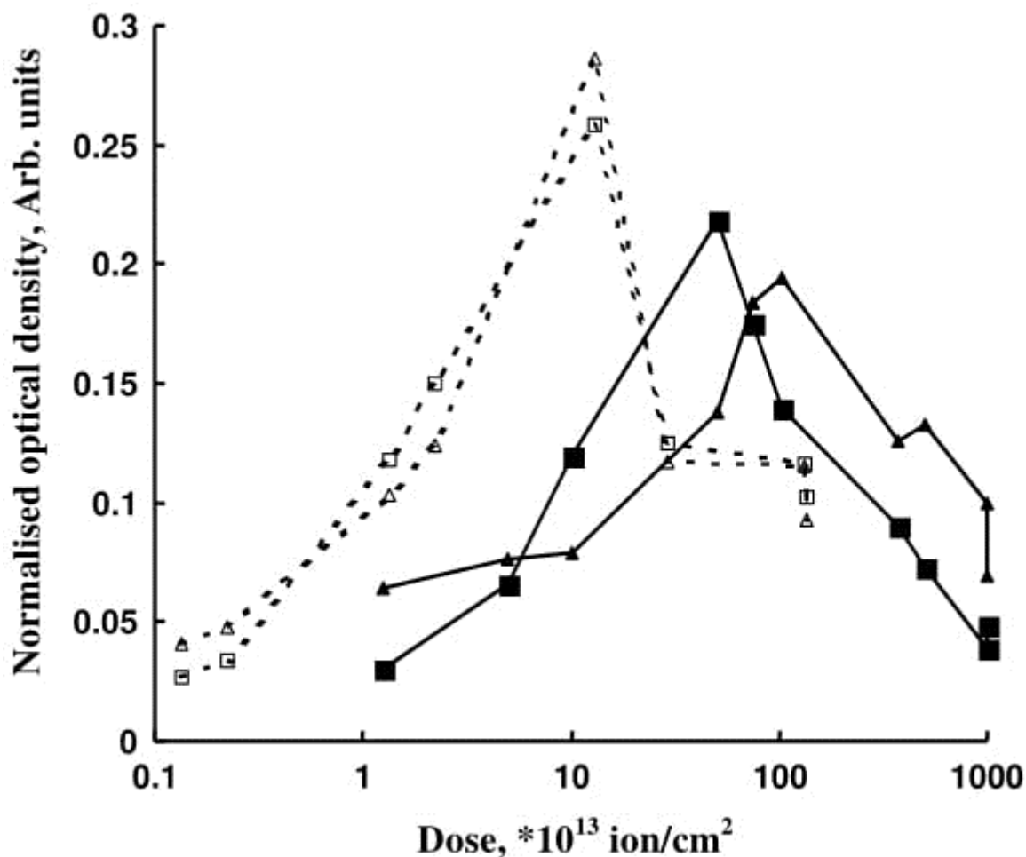
Slika 3.9: Ovisnost normalizirane optičke gustoće (normalizirana apsorpcija) karakterističnih skupina \nu(C = O) 1720\text{ cm}^{-1} linije (trokuti), \nu(C = C) 1610\text{ cm}^{-1} linije (kvadrati) u IR ATR spektru PE nakon kontinuiranog (puna linija) i pulsnog (točkasta linija) tretmana ionskim snopom. Vidimo veće vrhove apsorpcije kod pulsnog načina rada snopa te se ostvaruju za manje doze zračenja nego kod kontinuiranog. Iz više ovakvih vrhova (pulsnih ili kontinuiranih) moguće je odrediti ovisnost apsorpcije o dozi pomoću koje možemo odrediti ovisnost veličine tragova o elektronskoj zaustavnoj moći. [34]
