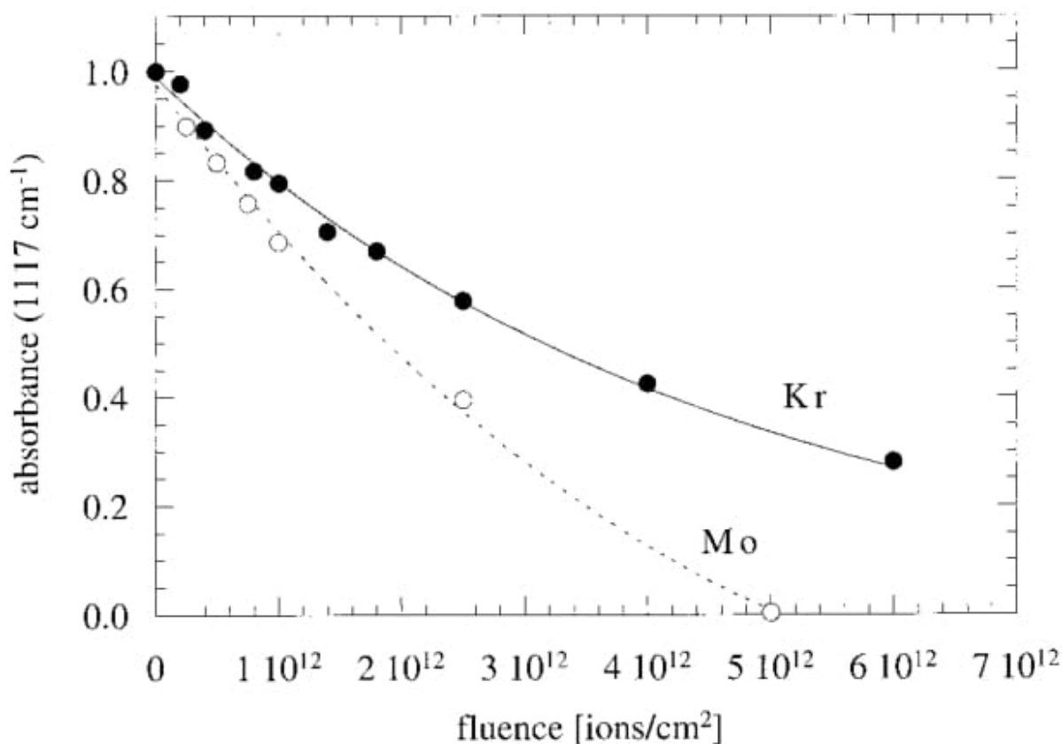
Slika 3.15: Normalizirana apsorbancija na vrpci 1117 \text{ cm}^{-1} koja pripada grupi CNC kao funkcija doze ionskog zračenja. Imamo ozračivanje ionima Kr u vakuumu i ionima Mo u atmosferi kisika. Vidimo značajniji pad apsorbancije kod ozračivanja Mo pa takvo mjerenje nije od koristi za procjenu dimenzije traga, dok je kod ozračivanja Kr izvjesna i saturacija što upućuje da je moguće sprovesti analizu. Iz grafa se može vrlo jednostavno procijeniti dimenzija traga. U ovom slučaju to je eksponencijalna prilagodba s općenitom konstantnom amplitudom gdje trag uz dozu \varphi u eksponent ulazi kao diferencijalni udarni presjek R^2\pi odnosno pretpostavljamo cilindrične tragove. [45]
