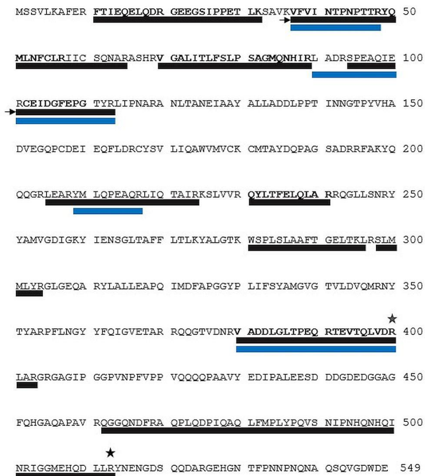
Slika 46. Peptidi detektirani u spektru PMF proteina NP u prugama u elutu E2 na slici 45. Crna linija – približna molekulska masa 57 kDa, plava linija – približna molekulska masa 45 kDa. Sekvencija peptida koji su sekvencirani MS/MS-om ispisana je podebljano. Strelice označavaju peptide koji su sekvencirani samo u jednoj prugi. Siva zvjezdica označava poziciju 400 koja skraćivanjem proteina s C-kraja daje protein od 45 kDa, a crna poziciju 513 koja skraćivanjem proteina s C-kraja daje protein od 57 kDa.
