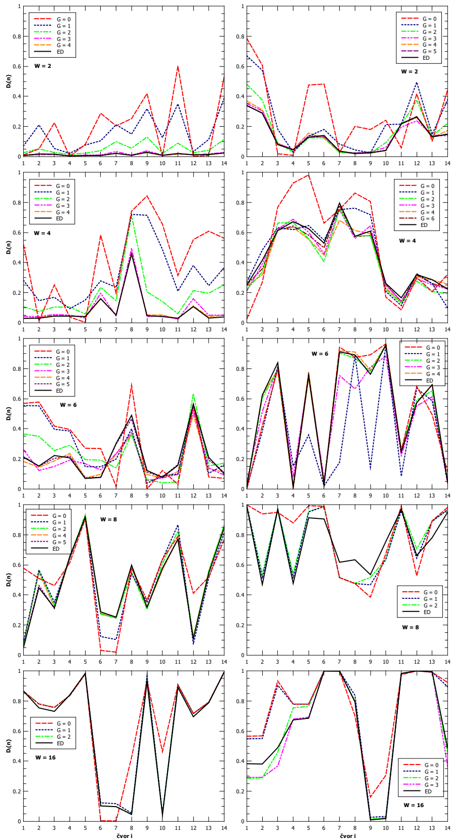
Slika 5.2: Krutosti gustoće naboja na pojedinom čvoru (5.12) izračunata unutar ARB za različite vrijednosti i konfiguracije nerada W = 2 - 16 . Uvjet rezonancije je postavljen na R^2 = 0.01 te G označava broj generacije. Dobiveni rezultati uspoređeni su s egzaktним vrijednostima (crna linija).
